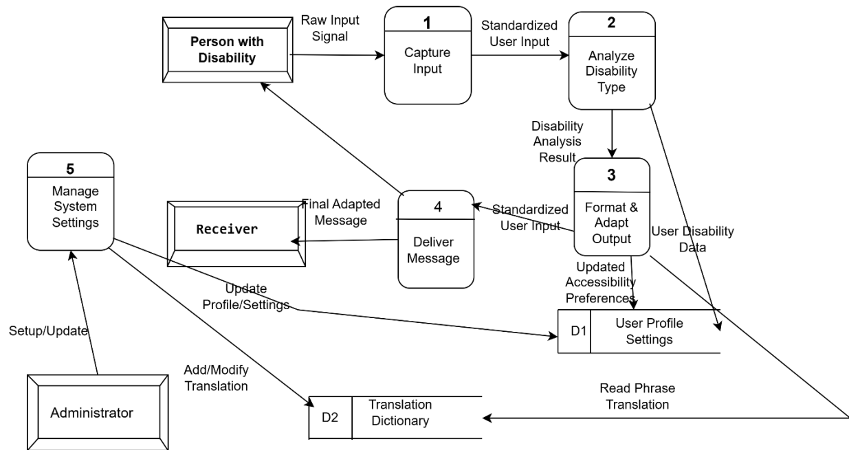
2.2.2.3 DFD (Level 2)
